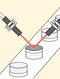
Rilevamento di un oggetto (tappo) capovolto Detecting the inverted caps
